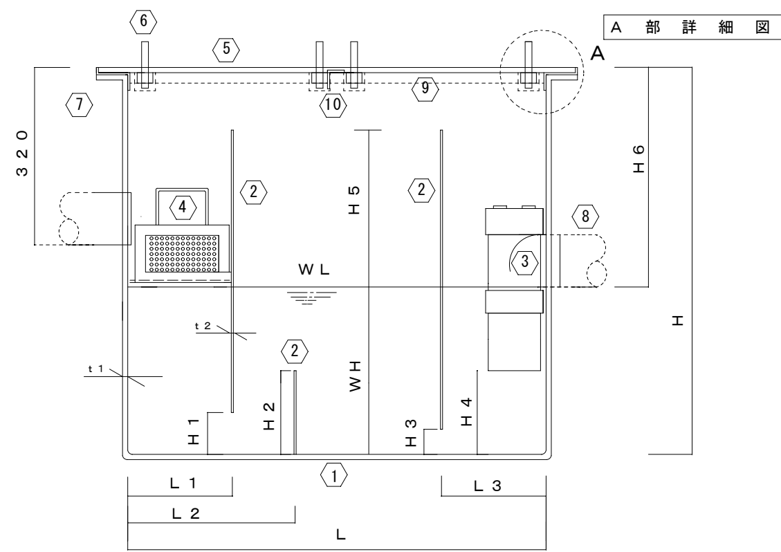
立面図
